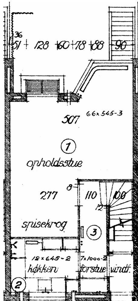
Stueplan
